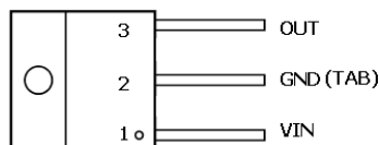
TO220-3L
