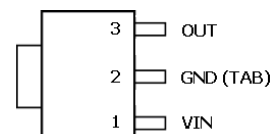
SOT223-3L
