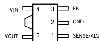
SOT89-5L
