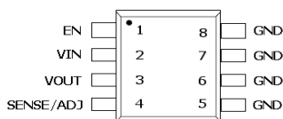
MSOP8
