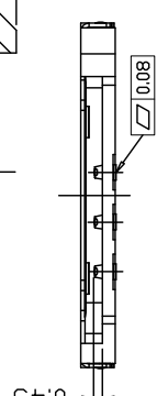
SECTION A-A
